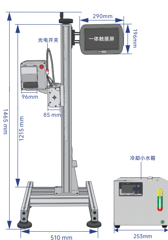
设备正面
