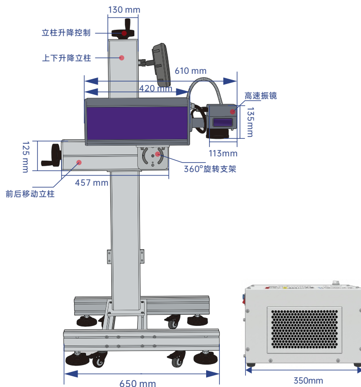
设备侧面
