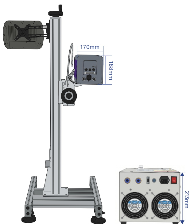
设备背面
